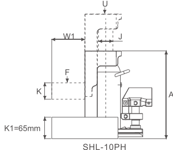
SHL-10PH
