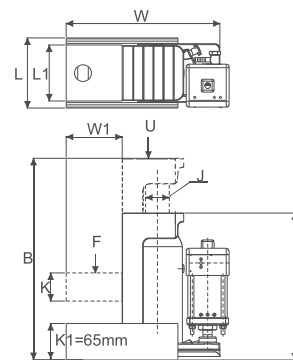
SHL-10P
