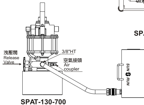
SPAT-130-700
